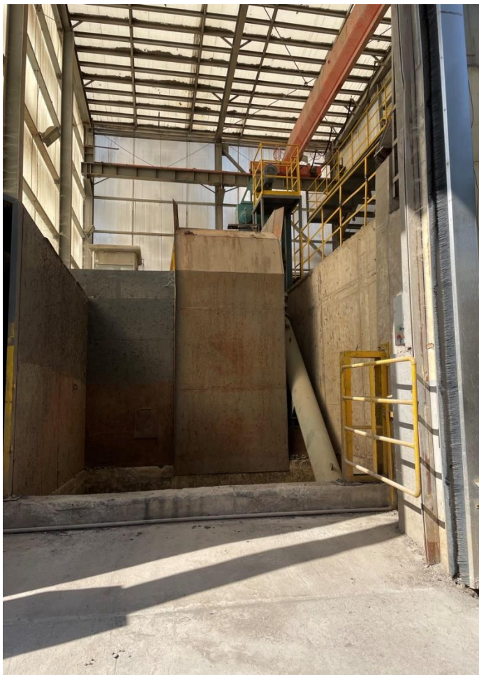
污泥仓
